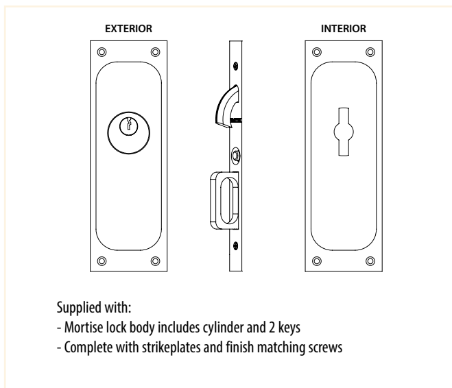
Passage Door Mortise Lock
